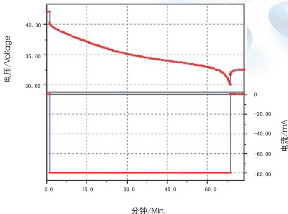
1C放电曲线图
