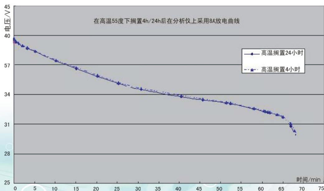
高温55°C 放电曲线
